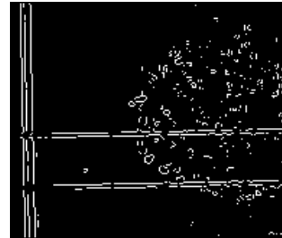
Edge Image
